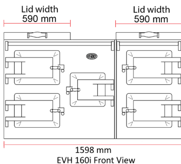
EVH160i dimensions
